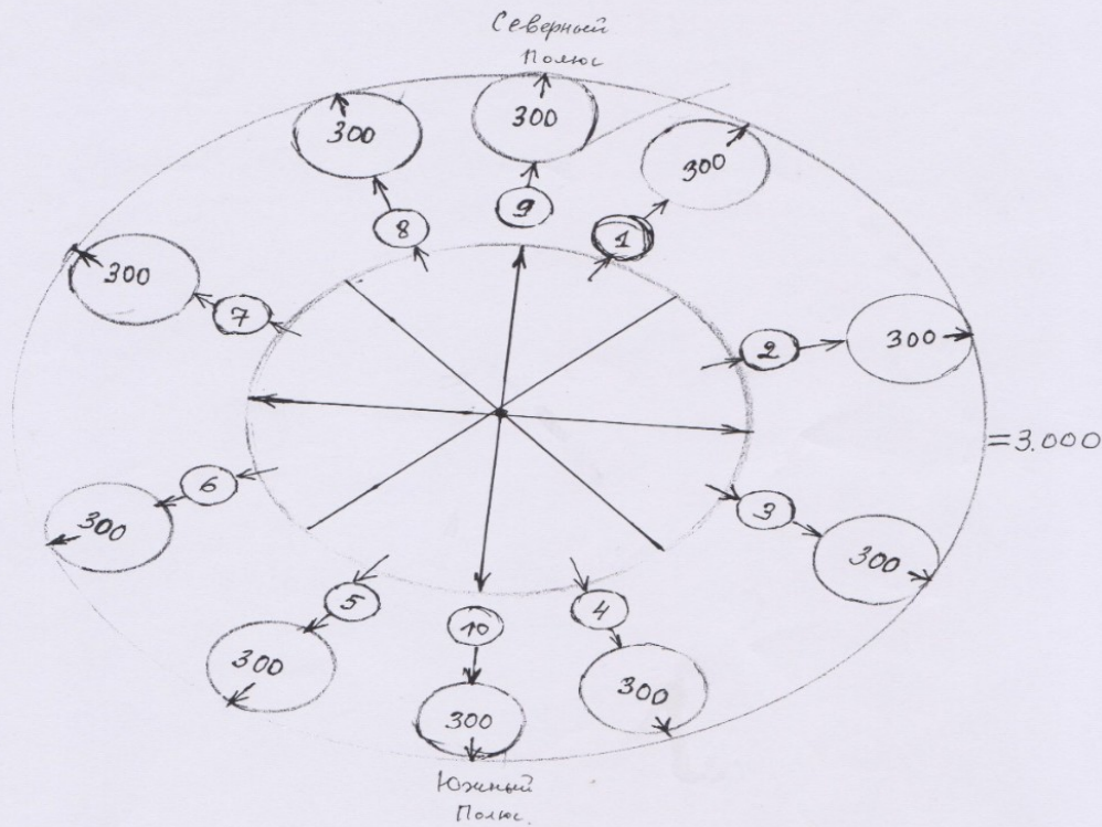
Схема сверхвселенной №1
